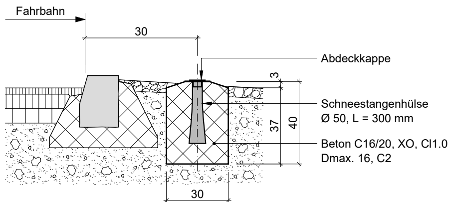
Bodenhülse mit Einzelfundament
