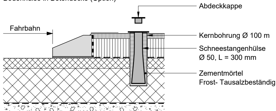
Bodenhülse in Betondecke (Option)
