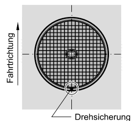
Grundriss Schachtabdeckung
