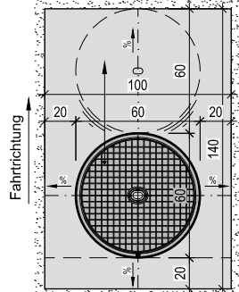
Grundriss Schachtabdeckung
