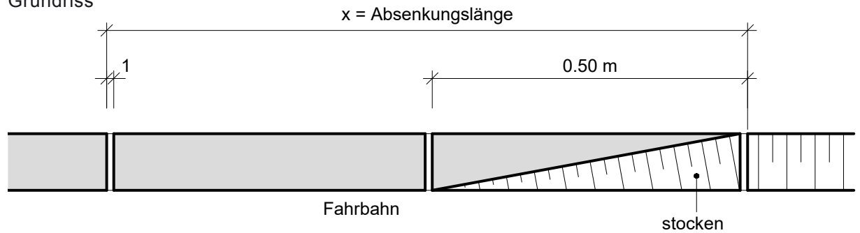
Grundriss
